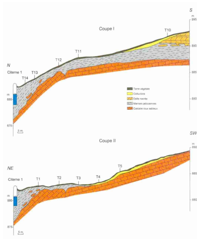
Coupe à travers le versant en amont de la citerne A. La coupe 1 révèle que la citerne est implantée dans les Marnes calloviennes, au bas d'un coteau constitué par cette même formation. La coupe 2 montre la relative proximité du fond de la citerne avec la roche calcaire en direction du sud-ouest. (MICHEL GUÉLAT, SÉDIQUA)
