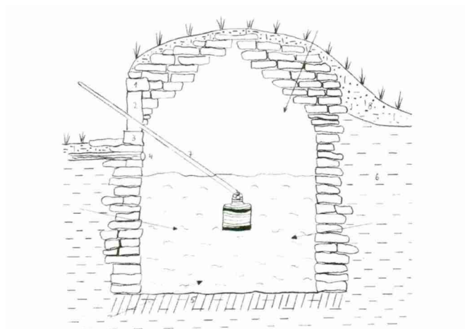
Coupe sur la citerne circulaire: 1-3. éléments constituant la porte, 4. trop-plein en bois, 5. couche de marne tassée, 6. couche de marne gorgée d'eau, 7. puisoir ou poujou, 8. terre végétale recouvrant la citerne (APCE, LUCETTE STALDER)
